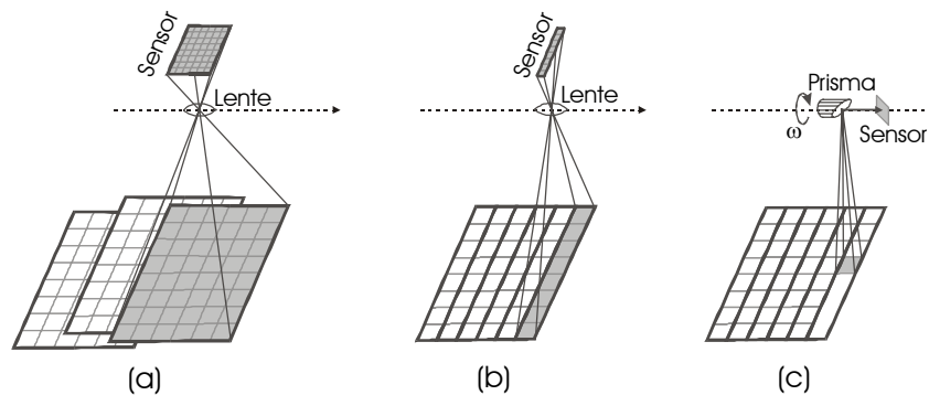
Figura 1: Geometría de los sensores digitales aerotransportados:
